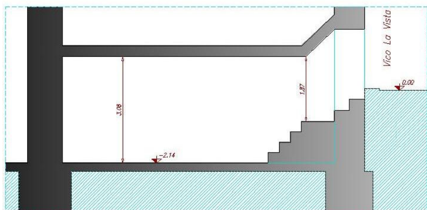
Sezione A_A
