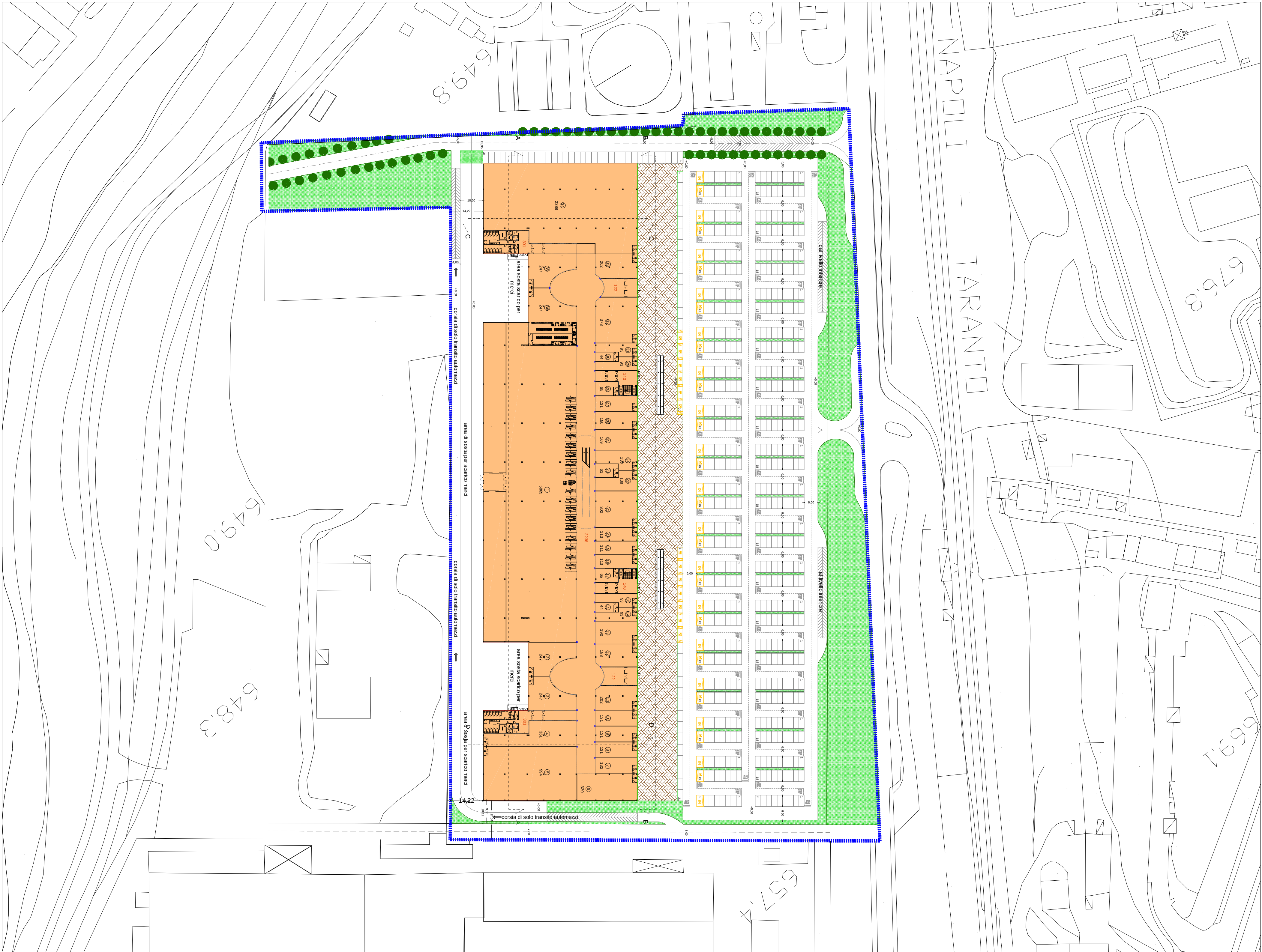
LIVELLO 0.00 - SCALA 1:1000
