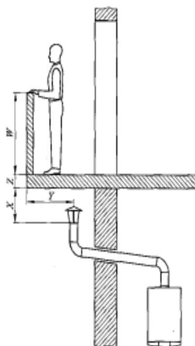
figura 6 Computazione percorso dei fumi
