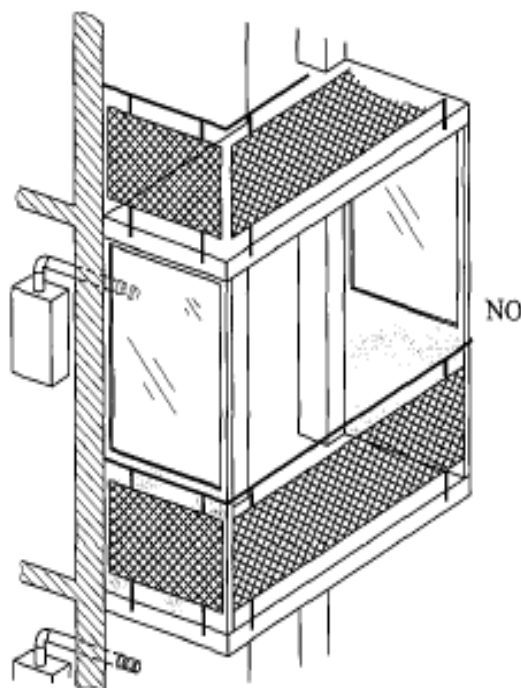
figura 13 Esempio di non corretta evacuazione dei prodotti della combustione all'interno di un balcone chiuso su cinque lati
