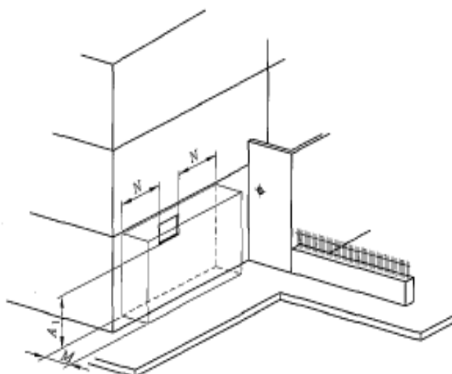
figura 9 Zona di rispetto di una finestra situata in una parete ortogonale a quella in cui è posizionato un terminale di tiraggio
