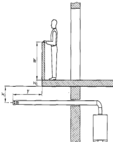
figura 12 Computazione percorso dei fumi con terminale sporgente il balcone
