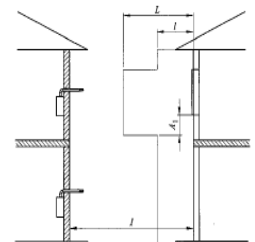
figura 14 Zona di rispetto di una parete (contenente un'apertura) frontale a quella in cui è posizionato un terminale di scarico
