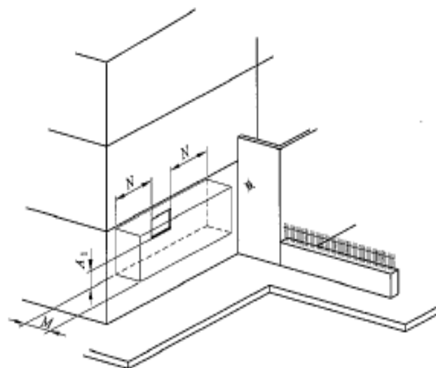
figura 15 Zona di rispetto di una finestra situata in una parete ortogonale a quella in cui è posizionato un terminale di scarico
