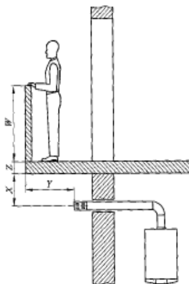
figura 11 Computazione percorso dei fumi
