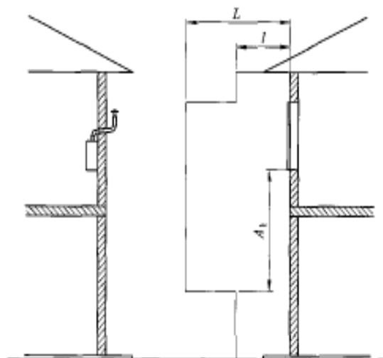
figura 8 Zone di rispetto di una parete (contenente un'apertura) frontale a quella in cui è posizionato un terminale di tiraggio
